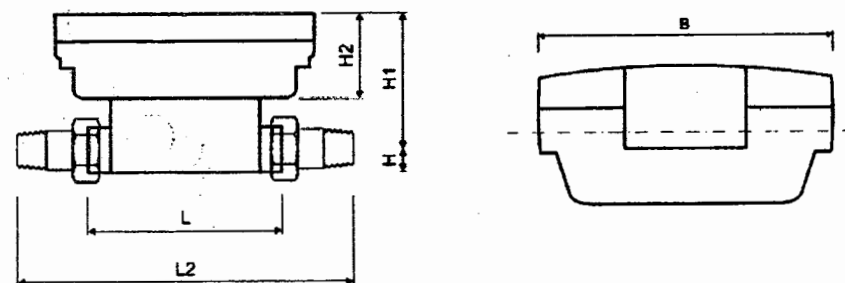
Рисунок 2 - Габаритные размеры теплосчетчика SHARKY с резьбовым соединением
