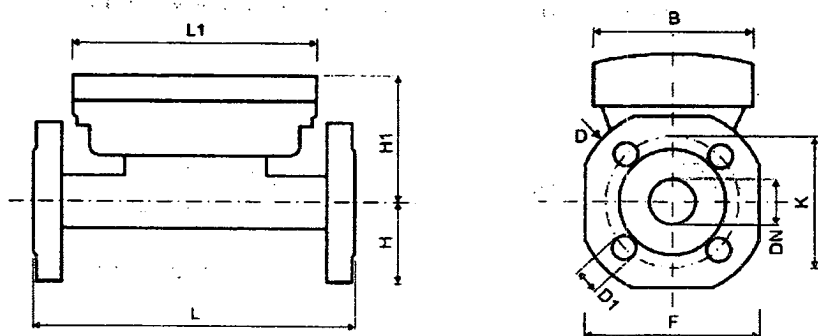
Рисунок 3 - Габаритные размеры теплосчетчика SHARKY с фланцевым соединением
