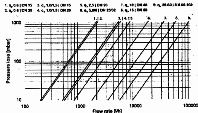
Рисунок 1 - Диаграмма потери давления теплосчетчика SHARKY
