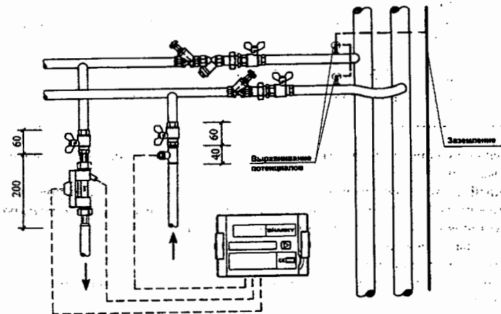
Рисунок 6. Схема системы выравнивания потенциалов на трубопроводах системы отопления.
