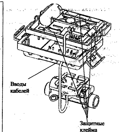
Рисунок C - Схема монтажа термопреобразователей сопротивления
