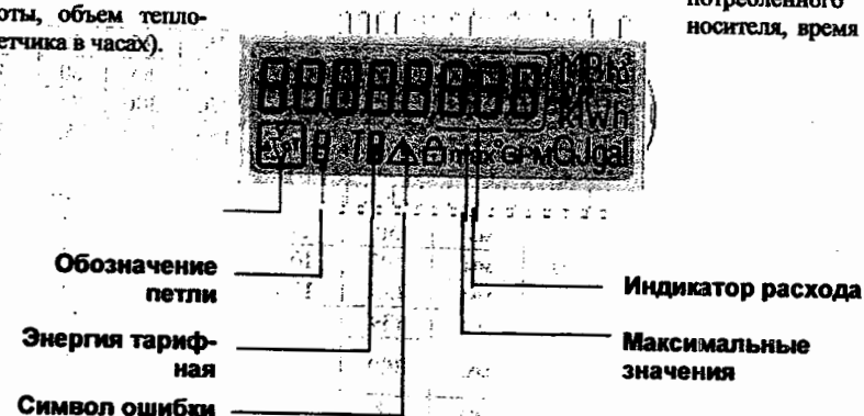
Рисунок 4. Схема дисплея вычислителя
