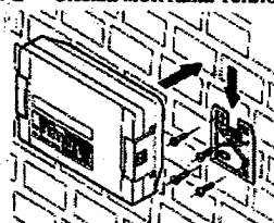
Рисунок F - Схема настенного монтажа вычислителя
